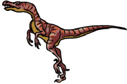
vélociraptor
