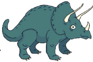
tricératops
